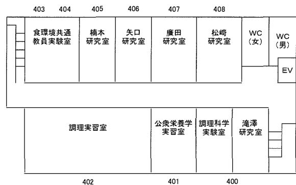
4 階 平 面 図
