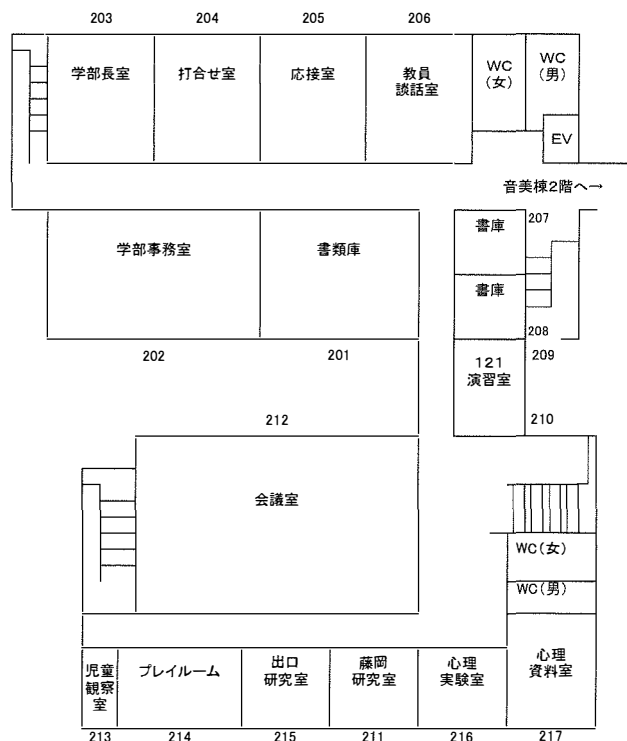
2 階 平 面 図
