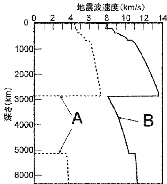
図1-3 地球内部でのP波とS波の地震波速度
