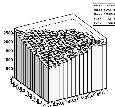
図2:余剰次元理論で予言される トップクォークのスピンの相関。 LHCで観測された場合の様子。
